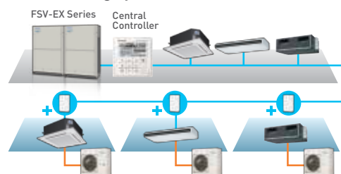
CZ-CAPRA1+CZ-CCERA1 H120×W70×D32.5mm
